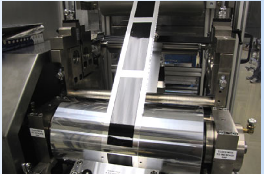
Pattern Die Coater
